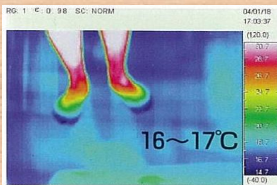
冬のリビングの床・一般住宅 (グラスウール 100mm)
